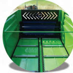
Çift sıra zincirli konveyör sistem Double row chain conveyor system
